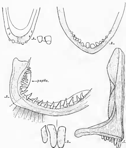
FIG. 8. — Paretroplus peliti (suite). A : Mandibule et 2 premières dents droite, face interne. B : Mâchoire supérieure. C : Mâchoire supérieure, vue latérale. D : Dents symphyséennes + dent gauche. E : 1 er arc branchial et papille.
